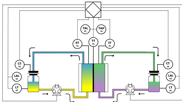
Figura 9. Diagrama P&ID sin válvulas.
