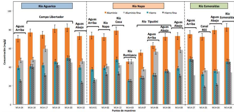
Gráfico 5: Concentraciones de Aluminio y Hierro en la fracción fina y en el bulk de sedimentos, en las cuencas de los Ríos Aguariño, Napo y Esmeraldas.
